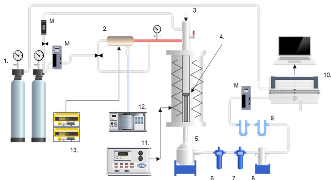
Зураг 2.7. Нүүрс хийжүүлэх туршилтын реактор
